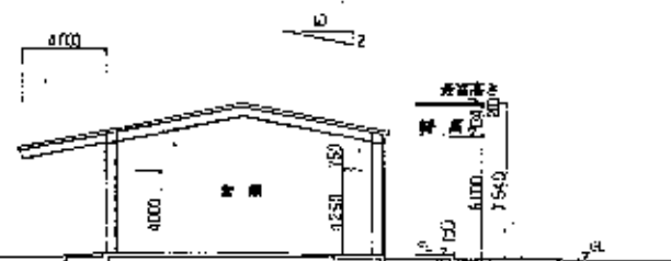
東立面図 S=1:200
