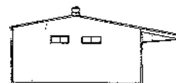
東立面図 S=1:200
