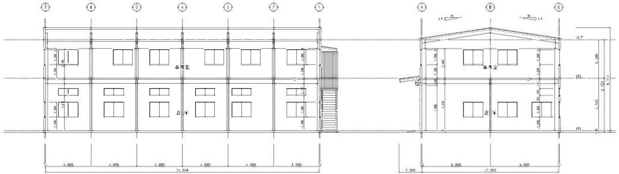
Y-Y 断面图 1:100
