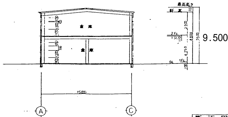
断面图 S=1:100
