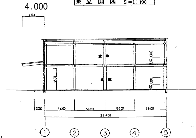
东立面图 S=1:100
