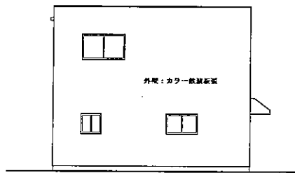
東側立面図 S 1:100
