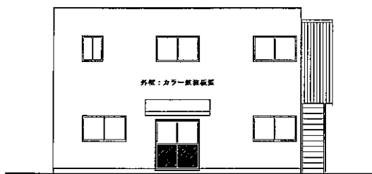
北側立面図 S 1:100
