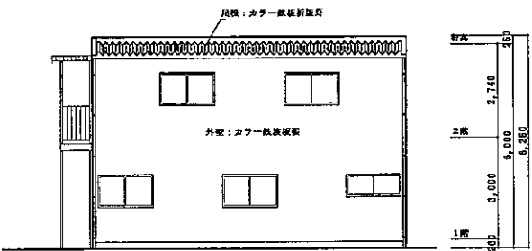
南側立面図 S 1:100
