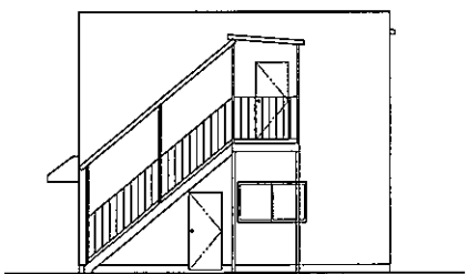
西側立面図 S 1:100
