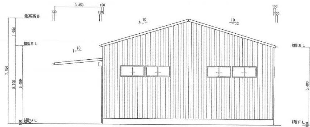
北側 立面图 S:1/100
