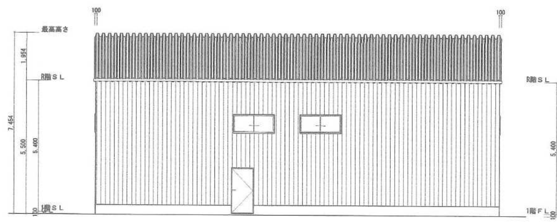
西側 立面图 S:1/100
