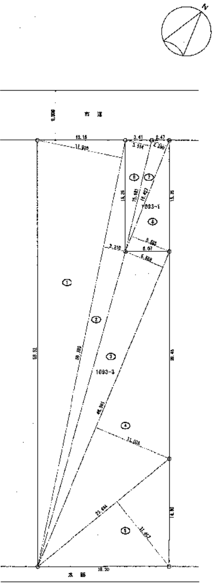
敷地求積図 S 1:250
