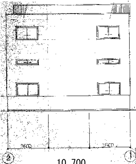
北側立面图 1/100
