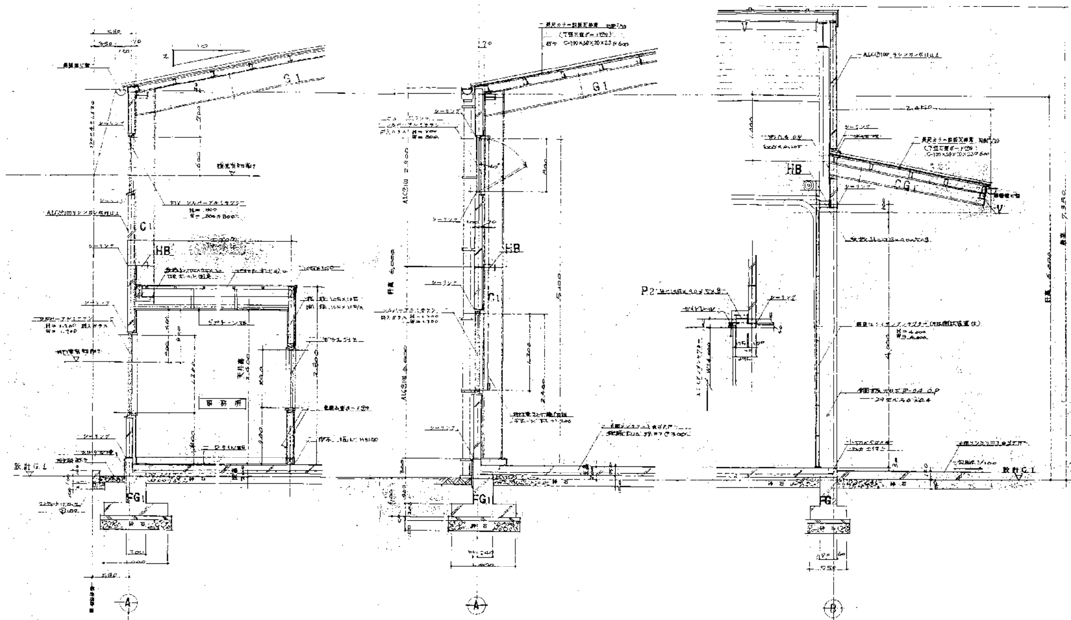
矩 計 図 S=1:30
