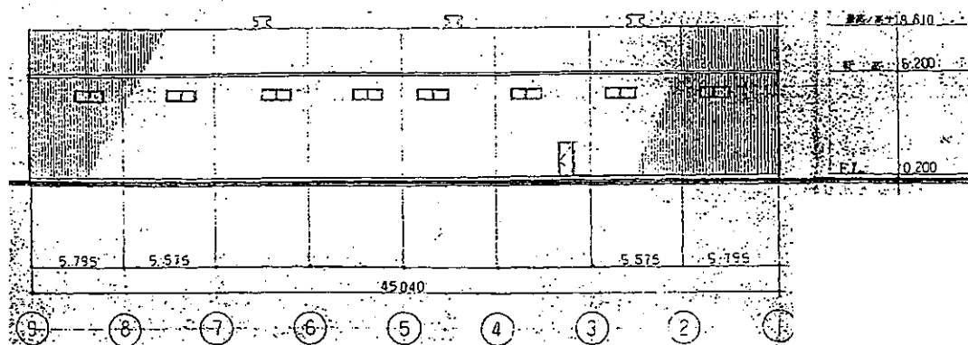
北立面图 S=1:200
