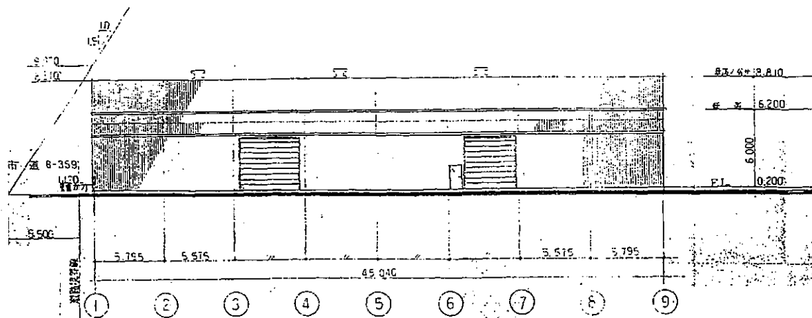
南立面图 S=1:200
