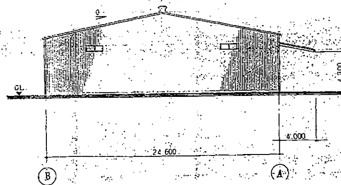
东立面图 S=1:200
