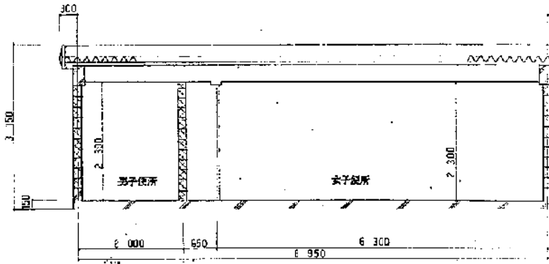
X-X 断面図
