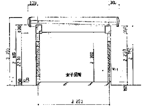
Y-Y 断面図
