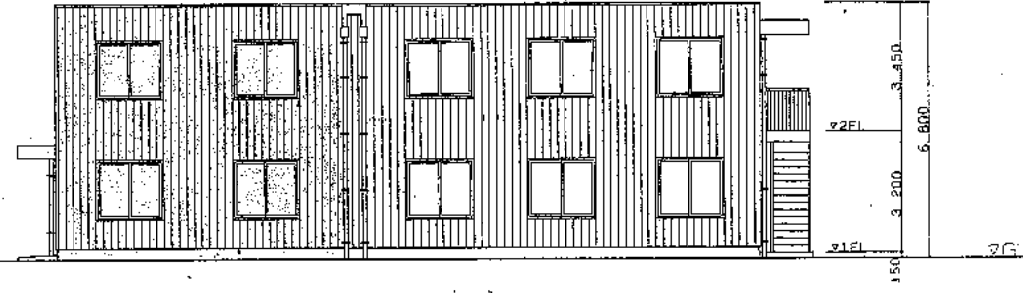
南立面図 S1:100
