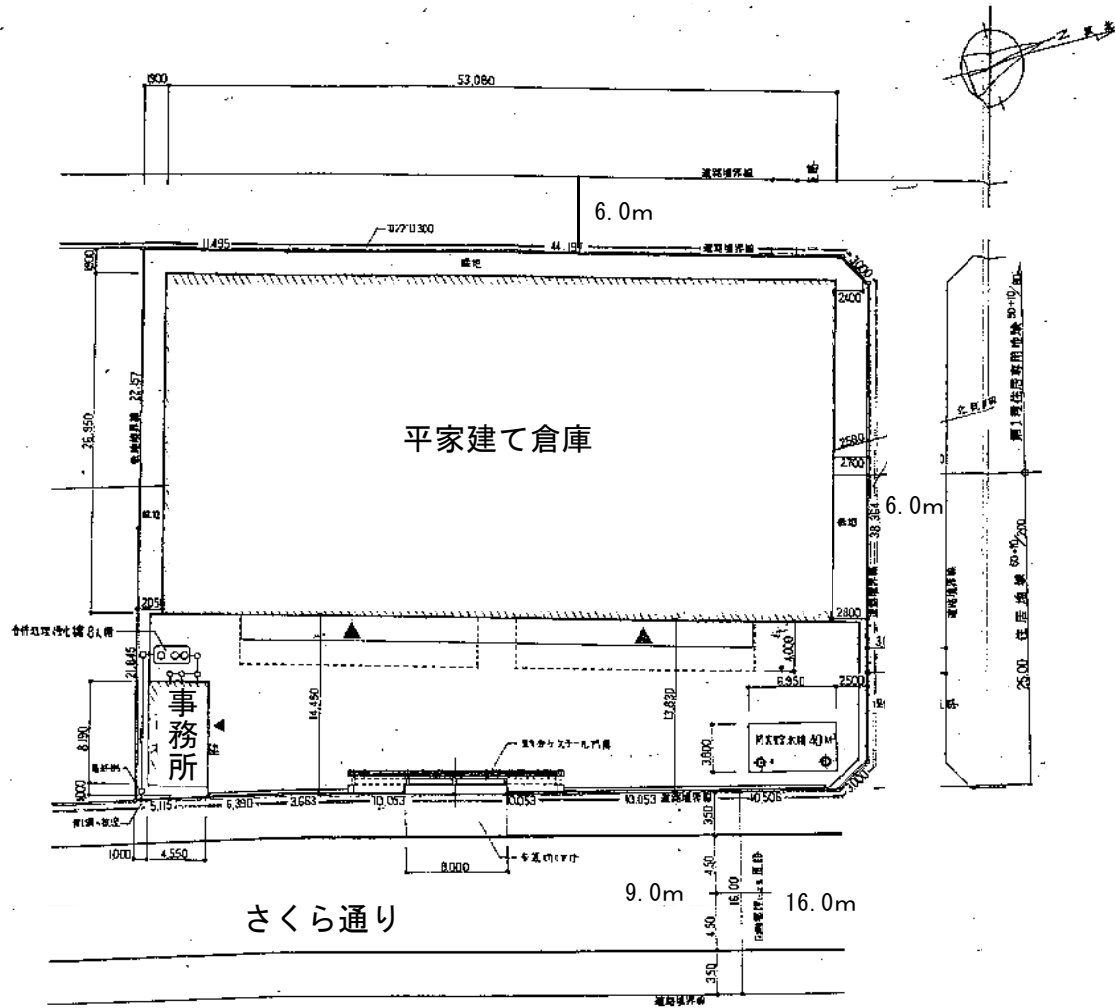
配置図 S=1:300
