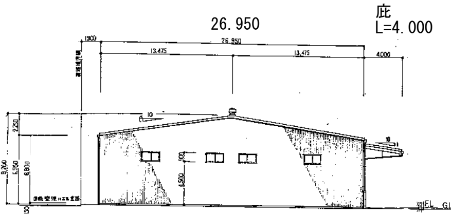
南面立面図 S=1:200
