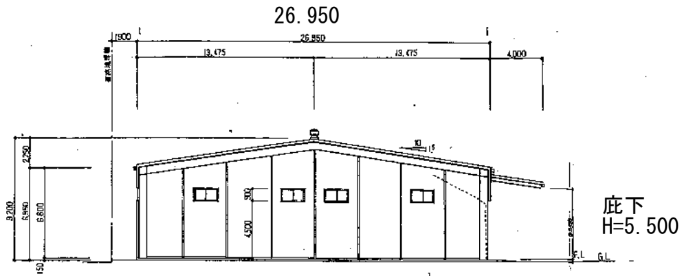
断面图 S=1:200
