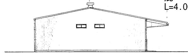
南立面图 S=1:200
