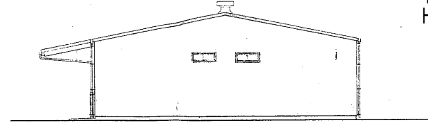
北立面图 S=1:200
