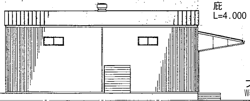
北立面図 S=1:100
