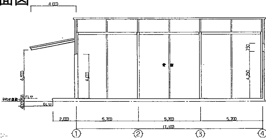
17.230 南立面図 S=1:100
