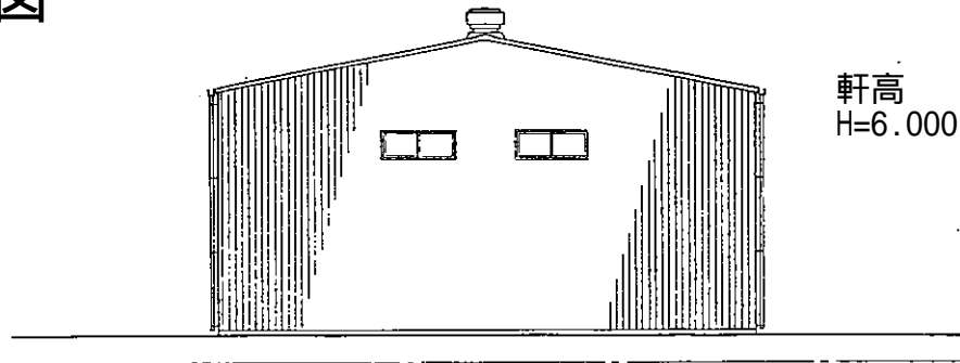
13.130 東立面図 S=1:100
