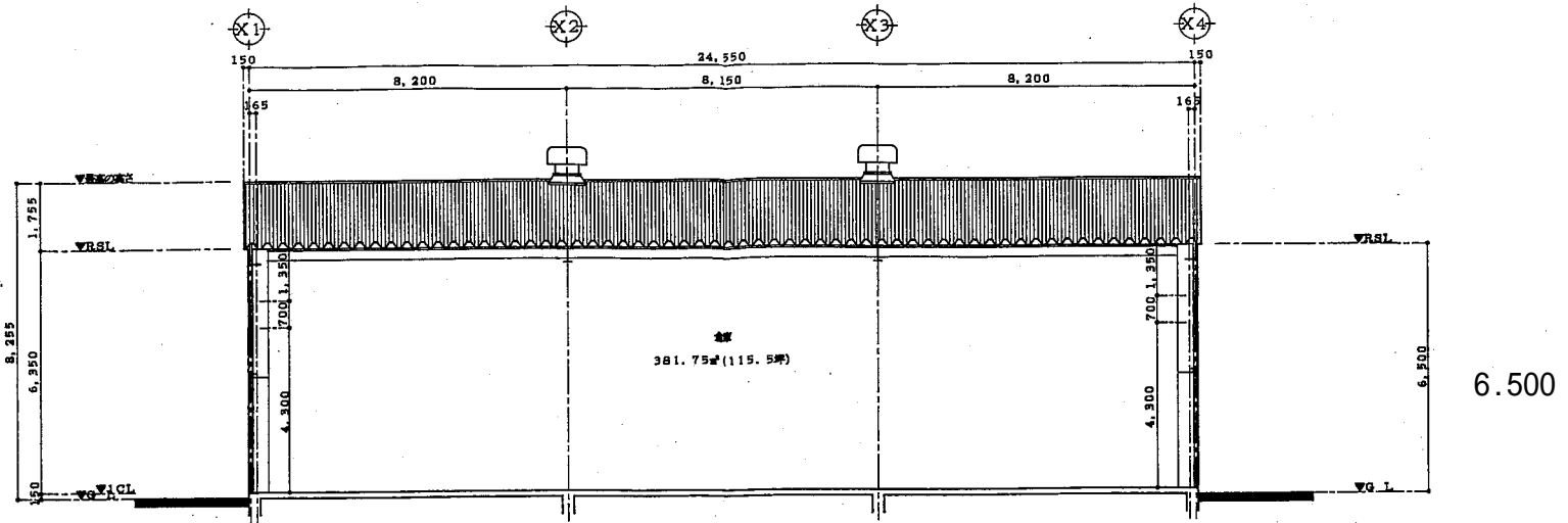
X-X 断面图
