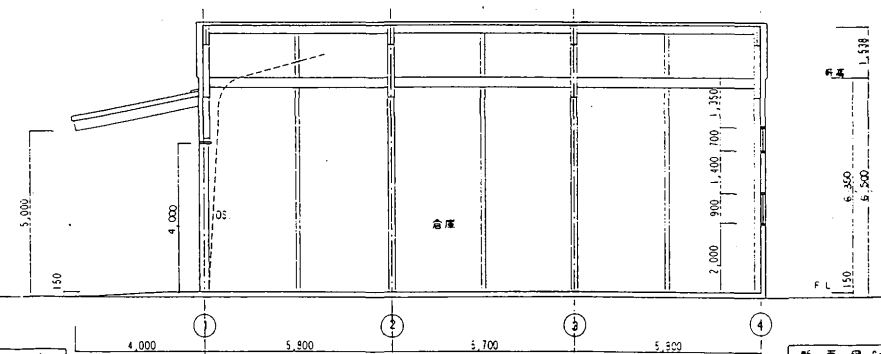
断面図 S=1/100
