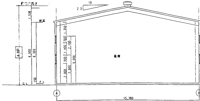
北立面図 S=1/100
