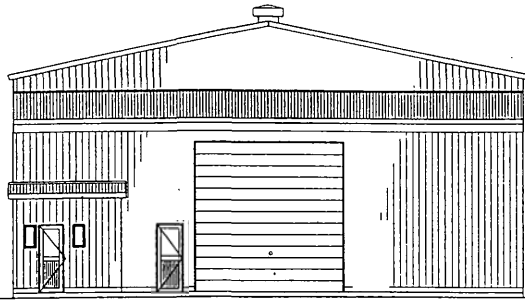
南立面図 S=1/100
