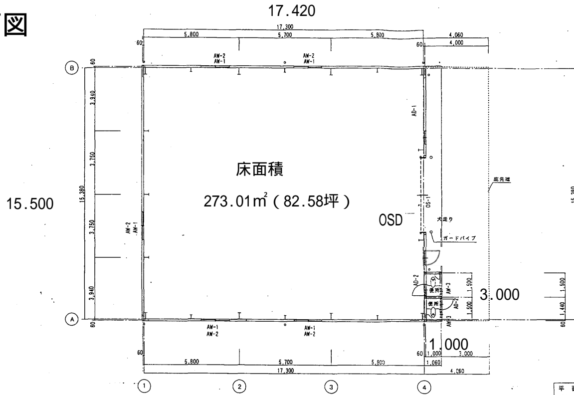
平面図 S=1/100
