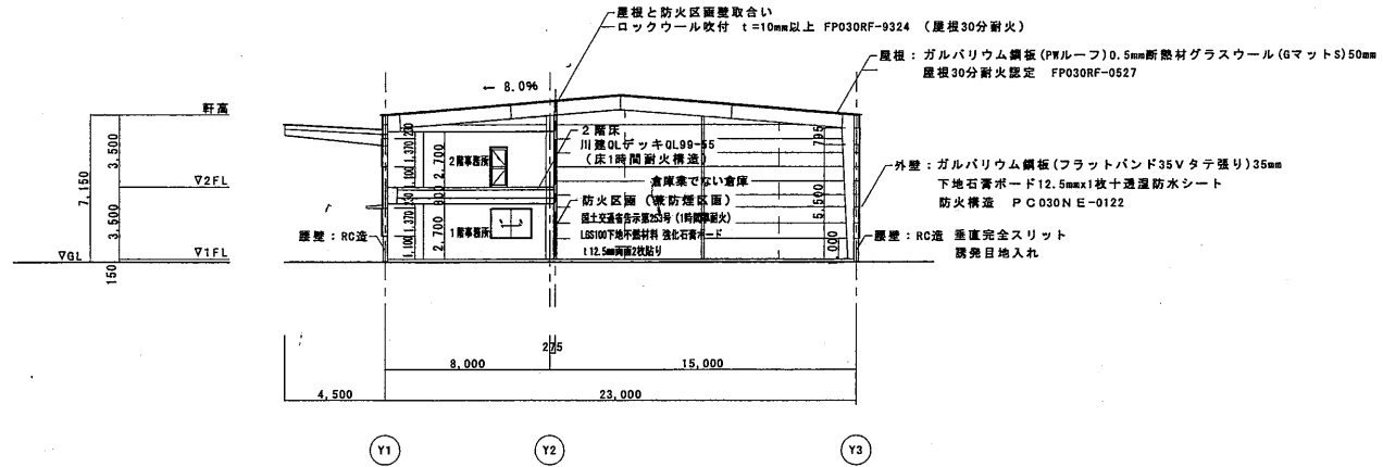
X2通り断面図
