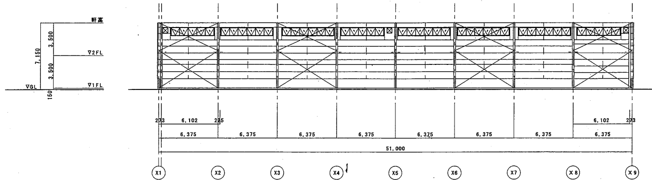
Y3通り立面図
