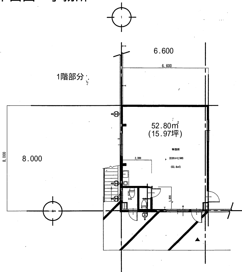
1階 平面図 S:1/200
