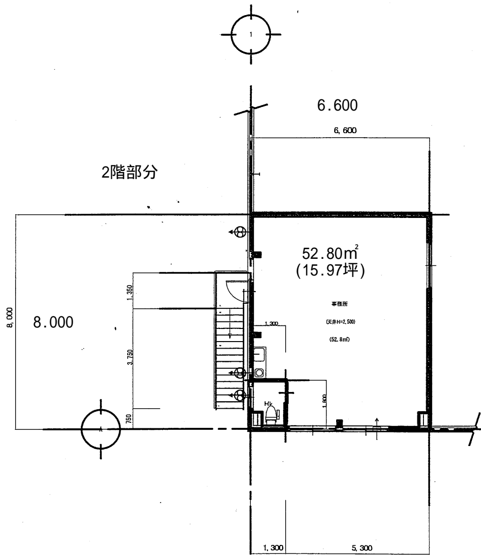
2階 平面図 S:1/200
