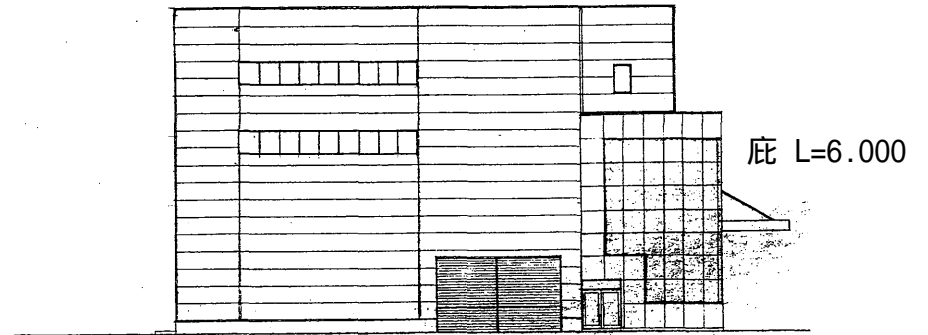
西立面図 S=1:200
