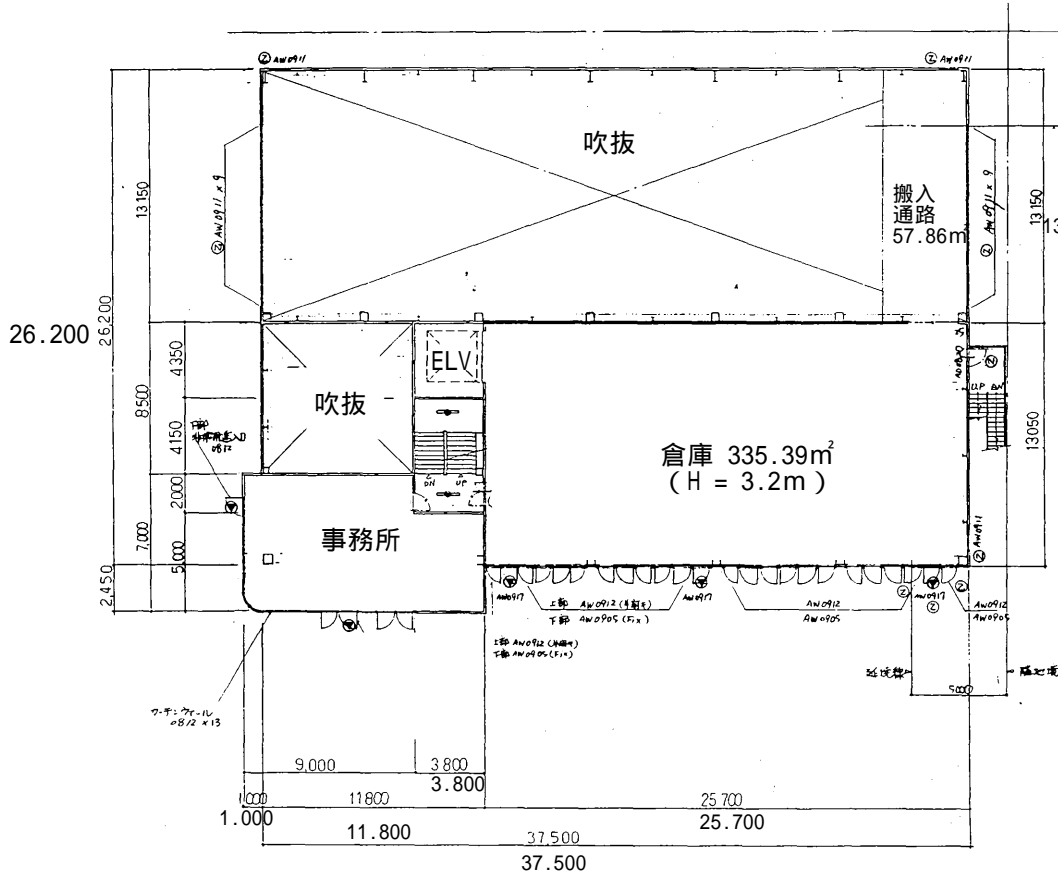
3階平面図
