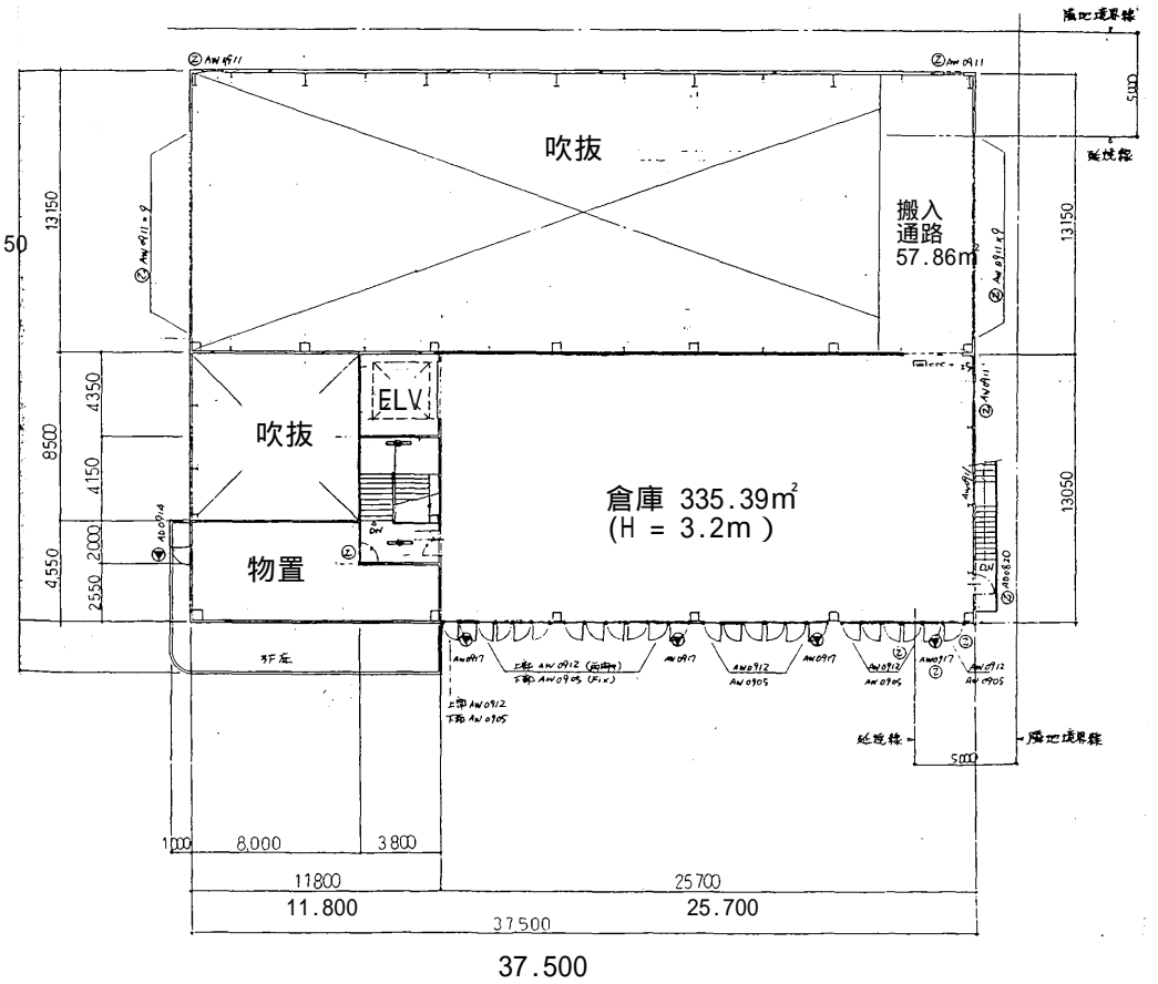
4階平面図
