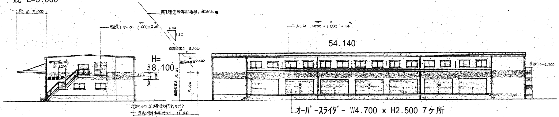
東立面図
