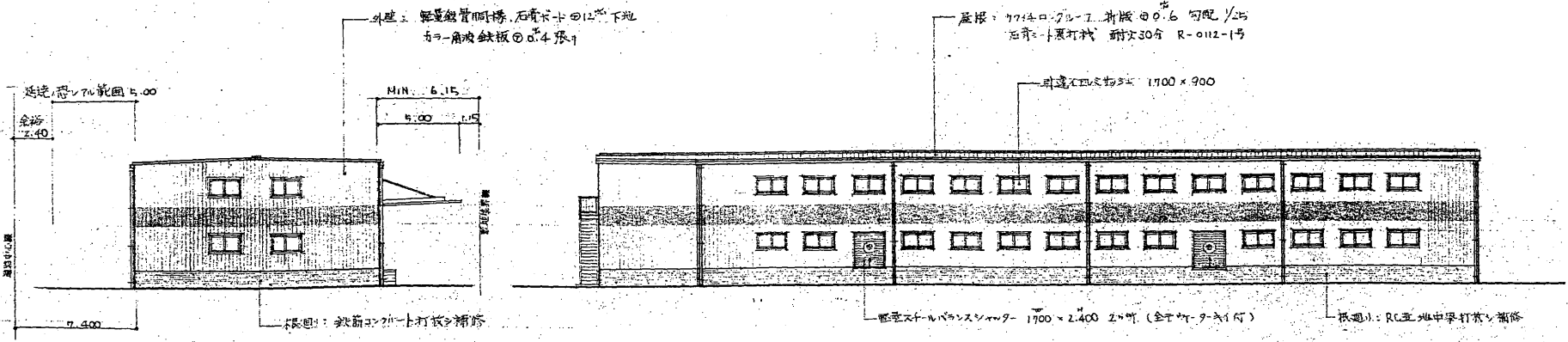
西立面図
