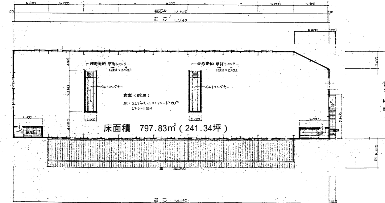
2階平面図
