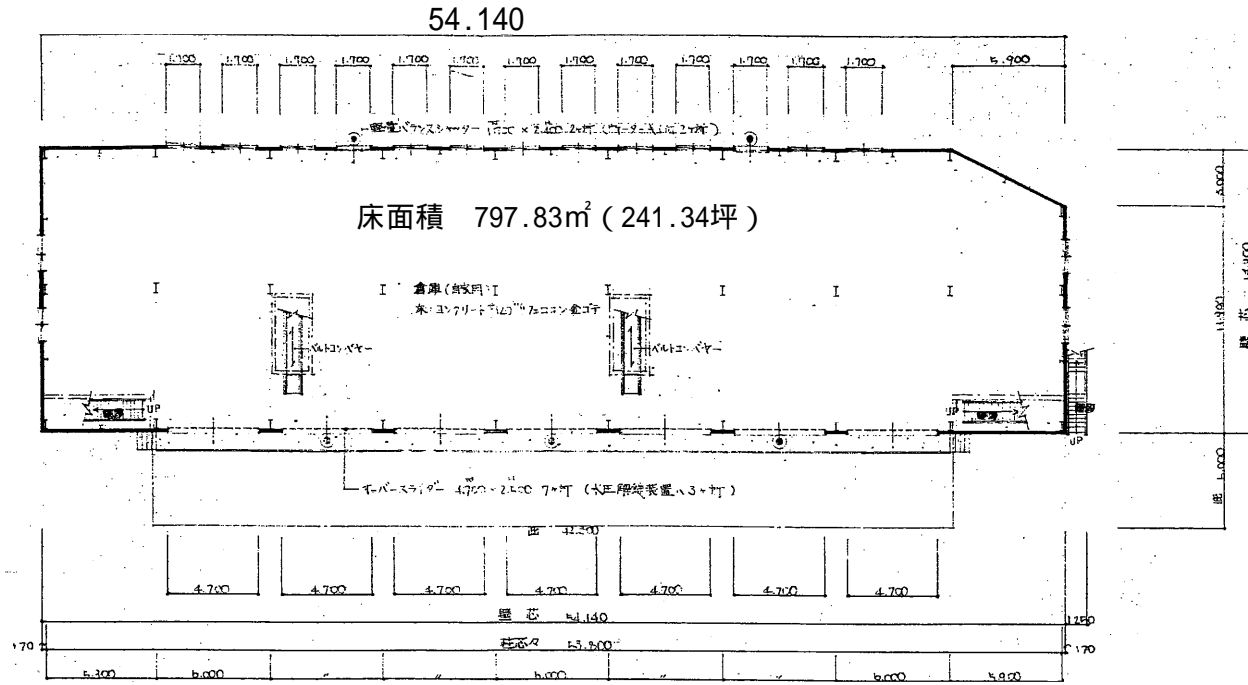
1階平面図
