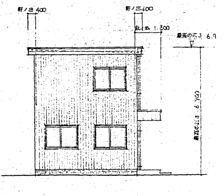
北立面図 S=1:100
