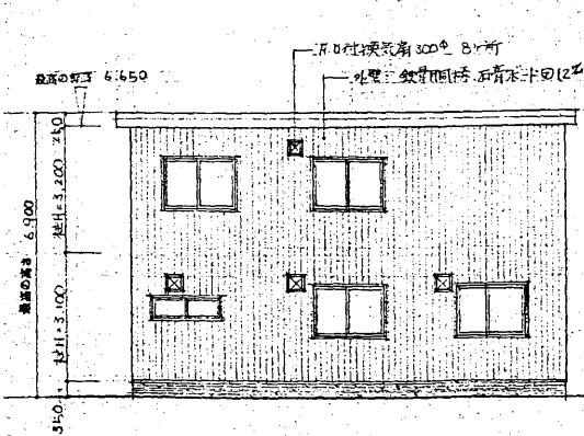
東立面図 S=1:100
