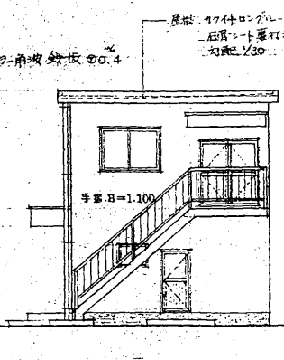
南立面図 S=1:100
