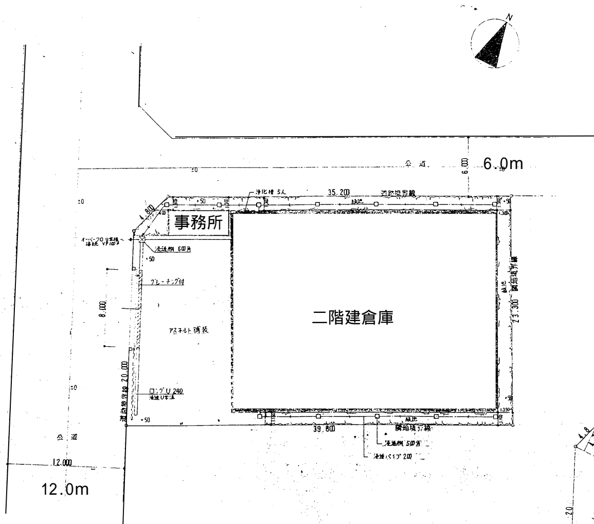
配置図 S=1/200 (排水系統図)
