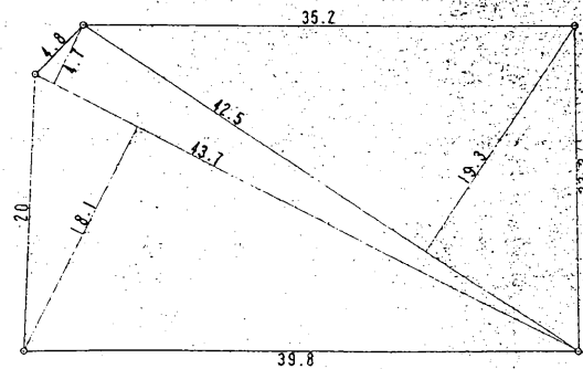
求積図 S=1/300
