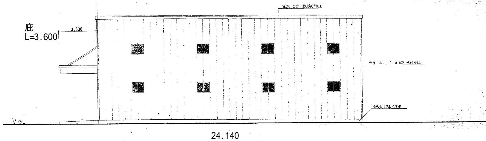
(南) 立面図 S=1/100
