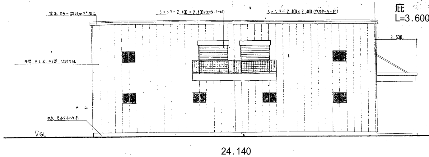
(北) 立面図 S=1/100
