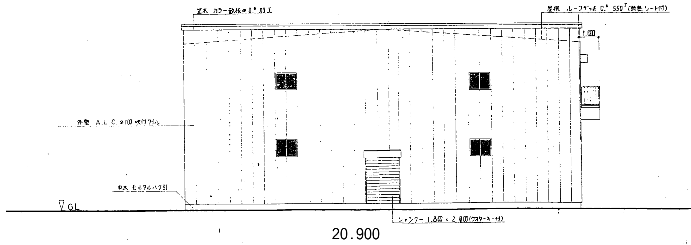
(東) 立面図 S=1/100
