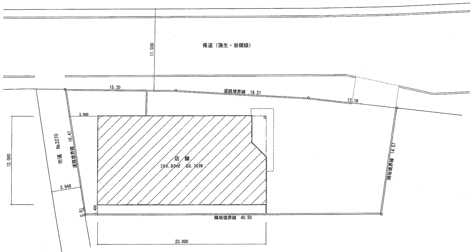
配置図 S 1:200
