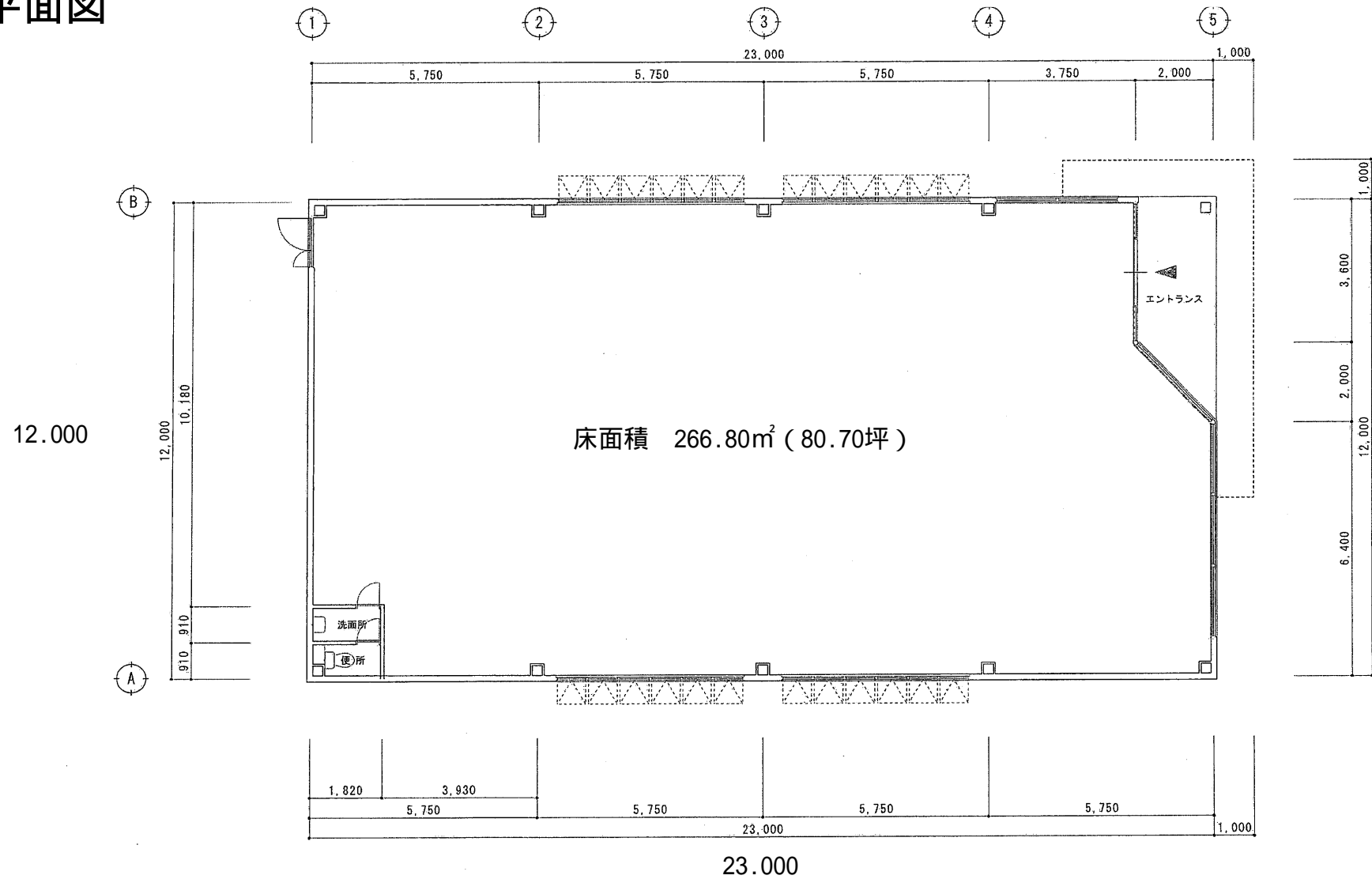
平面図 S 1:100
