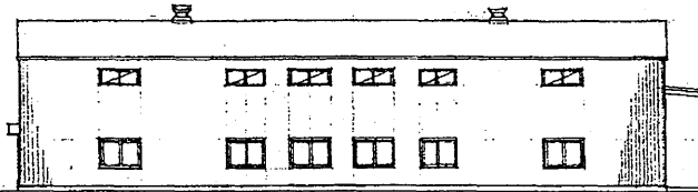
北立面図 1:200
