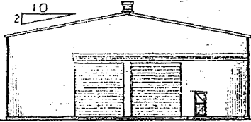
西立面図 1:200
