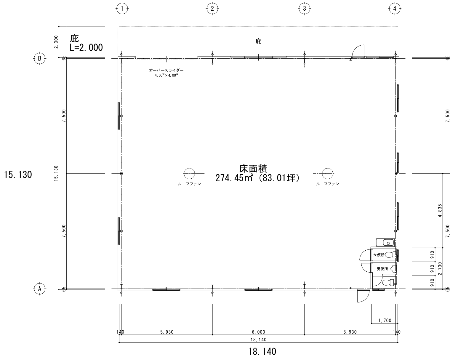
平面図 S 1:100
