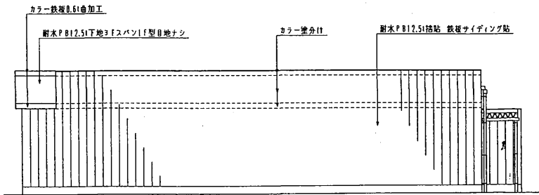
南立面図 1/100
