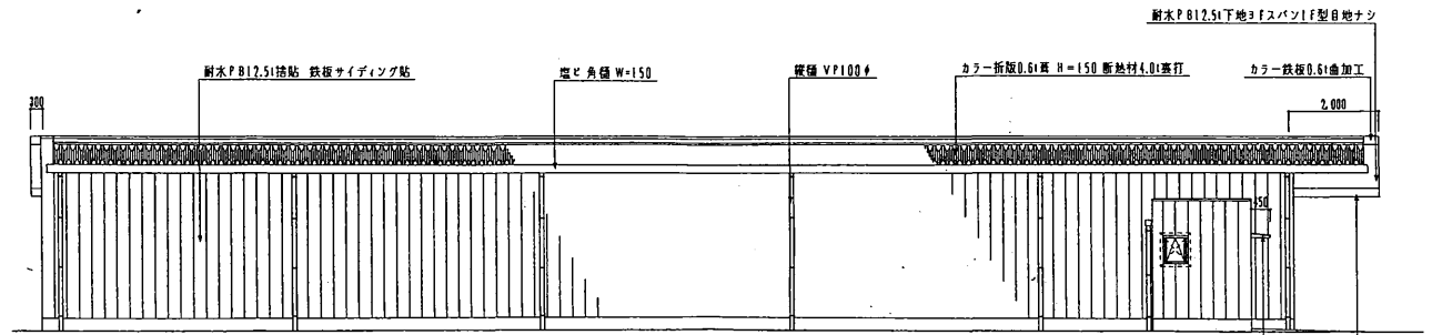
西立面図 1/100
