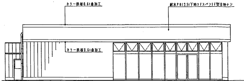
北立面図 1/100
