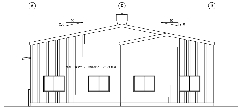
8.050 8.050 東側立面図 S 1:100
