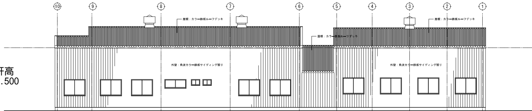
21.290 2.900 13.000 北側立面図 S 1:100
