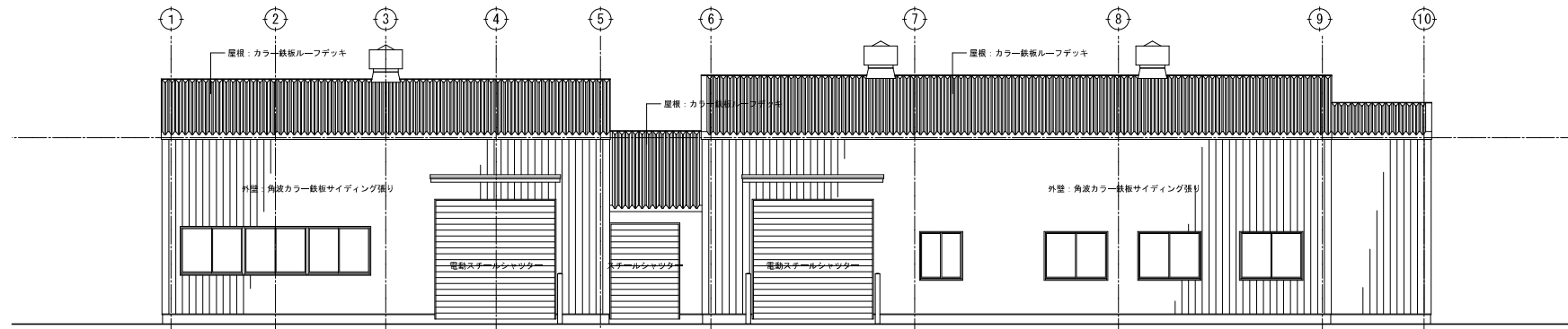
W3.500 H3.500 W2.000 H2.800 南側立面図 S 1:100
