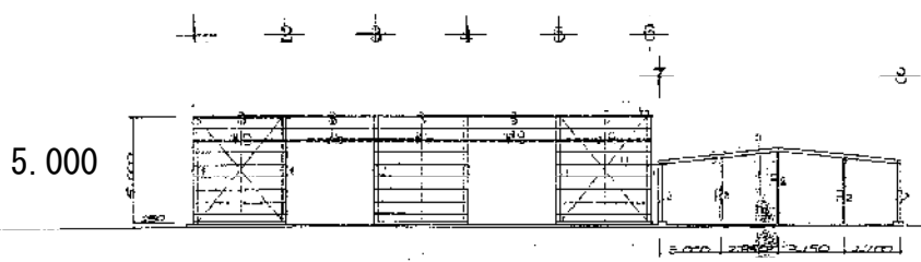
5 通 軸 組 圖 1/200
