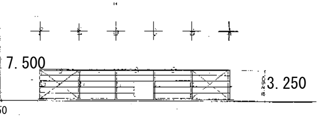
7 通 軸 組 圖 1/200
