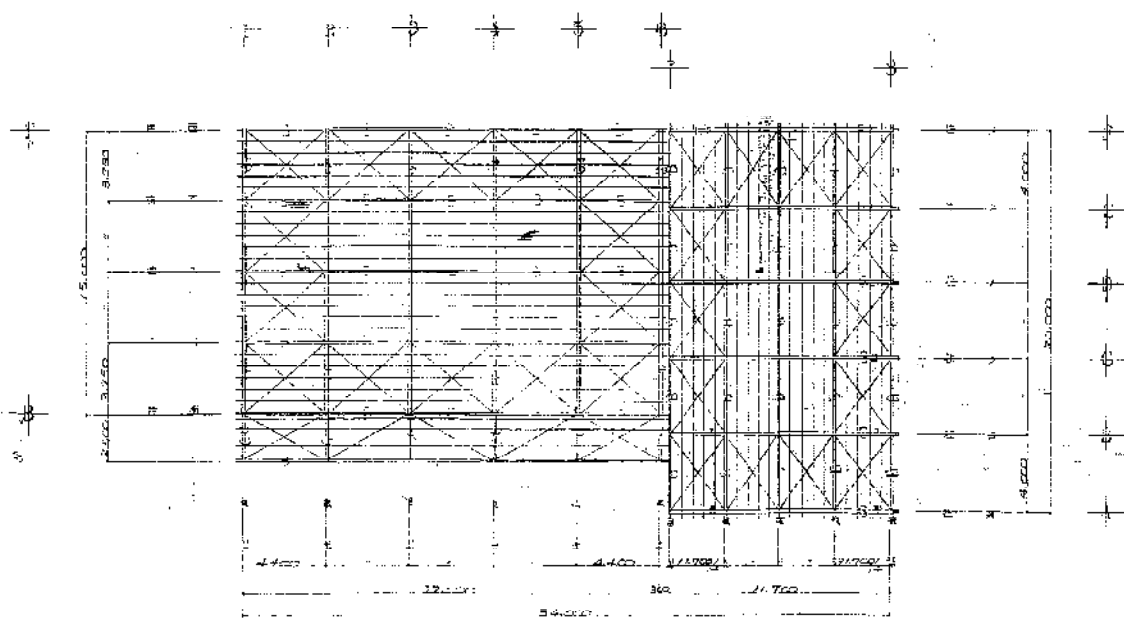
小 屋 屋 架 圖 1/200
