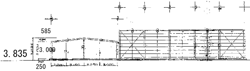
1 通 軸 組 圖 1/200
