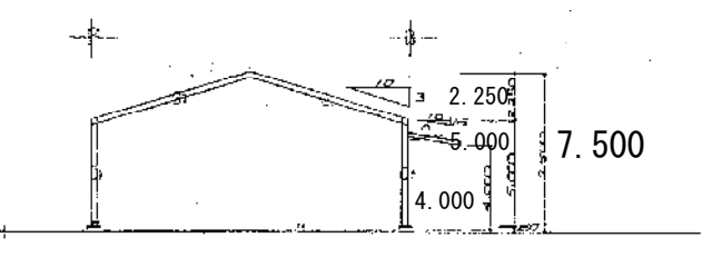
7~8 通 軸 組 圖 1/200
