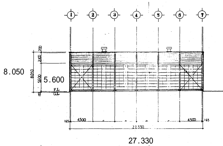
横断面図
