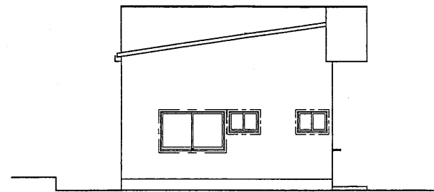
西 立面図 S=1/100
