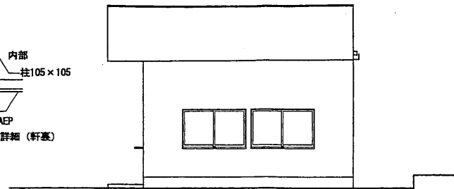
5.460 東 立面図 S=1/100
