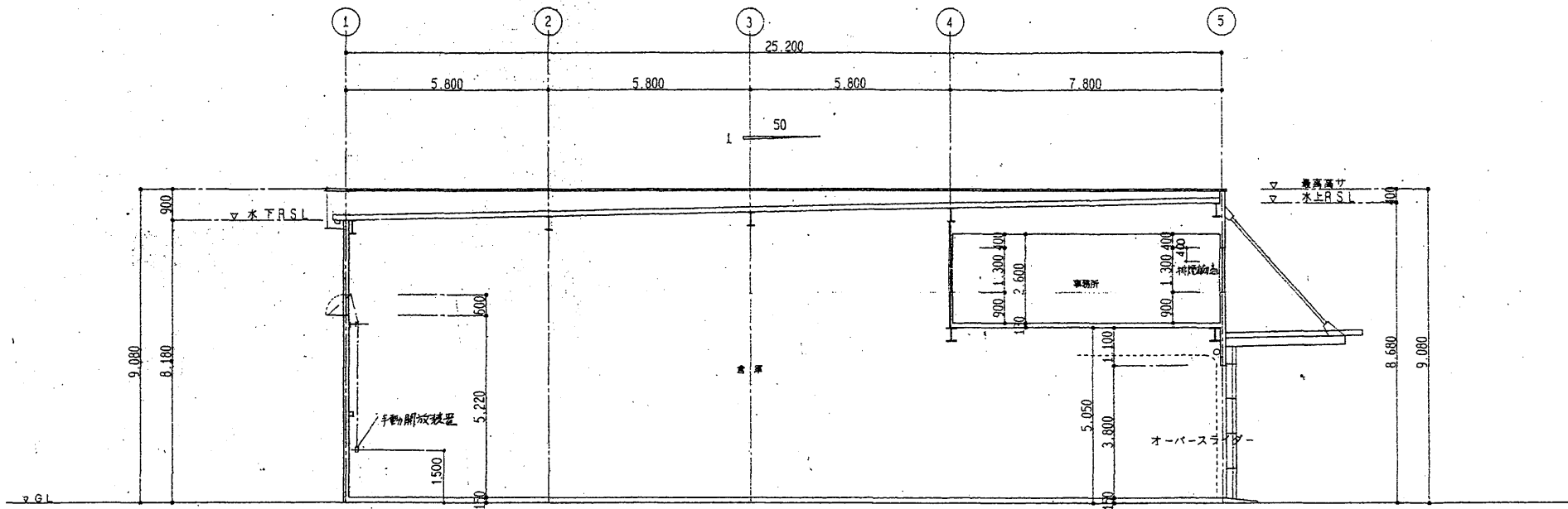
断面図 1 : 100
