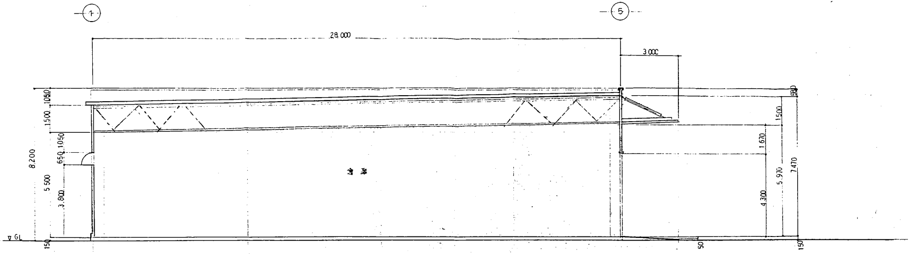
断面图 1/100
