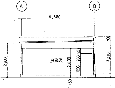
断面图 1/100
