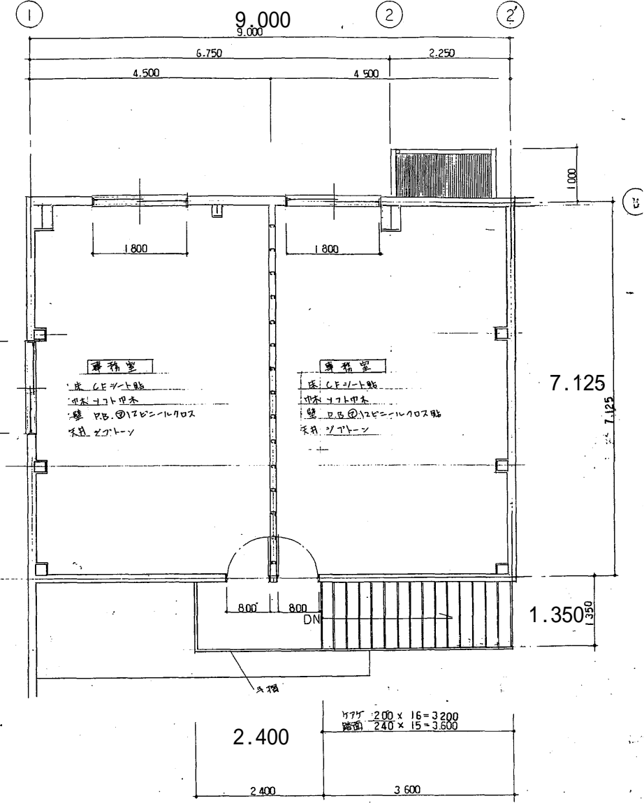
2階事務所部 平面詳細図 1/50
