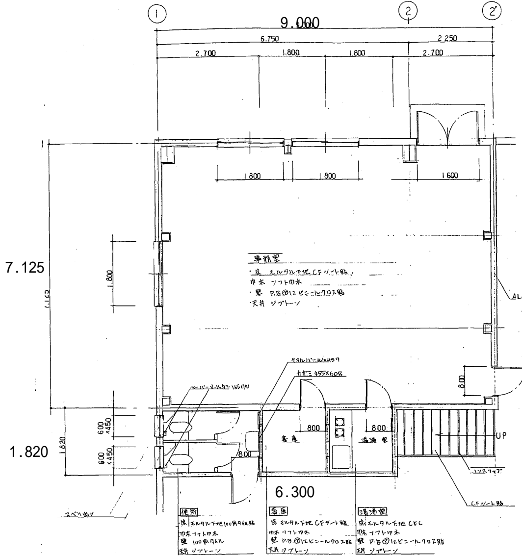
1階事務所部 平面詳細図 1/50
