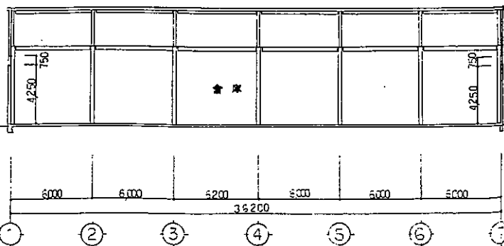
断面图 比例 1:200
