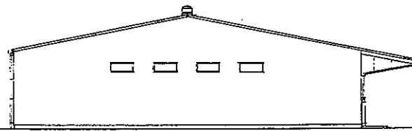
西立面图 比例 1:200
