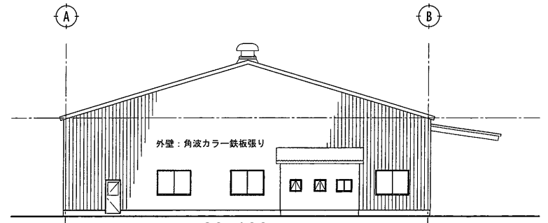
西側立面図 S 1:200
