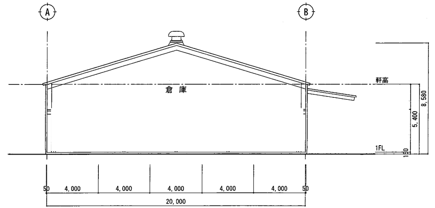
X-X 断面図 S 1:200
