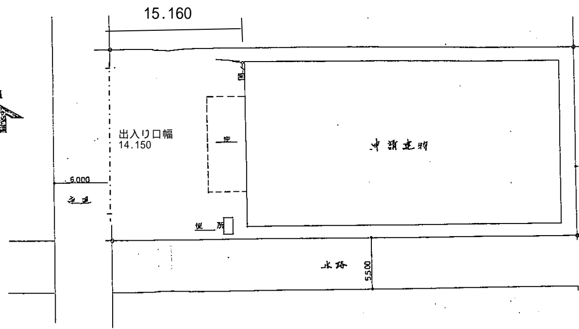
配置図 S=1:200
