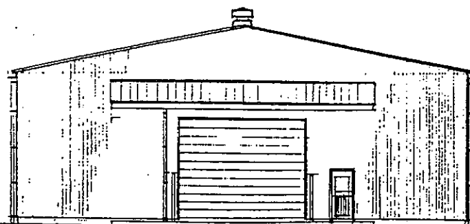
北立面図 S=1/100
