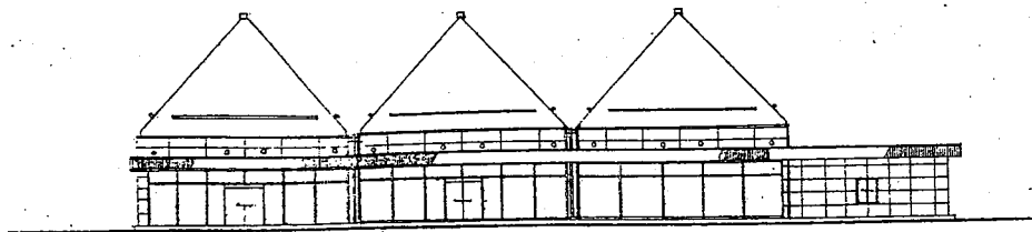
西立面图 1:200
