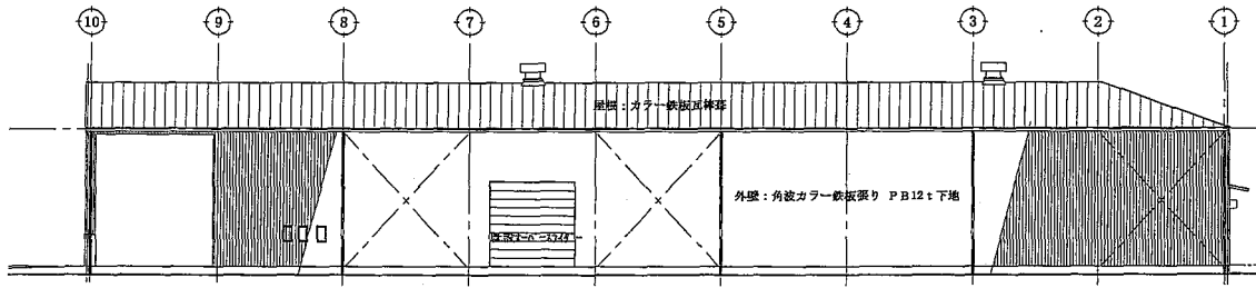
東側立面図 1: 200
