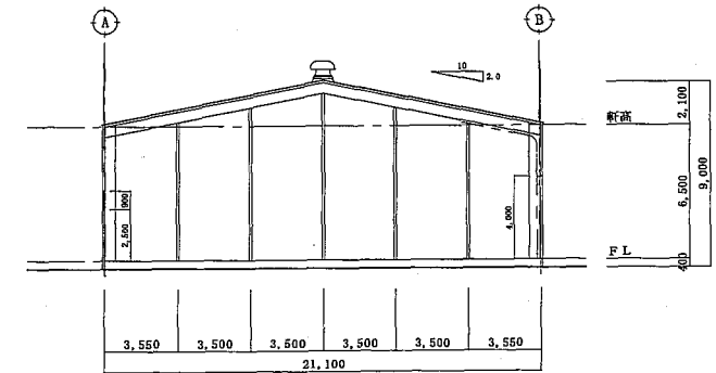
断面図 1: 200
