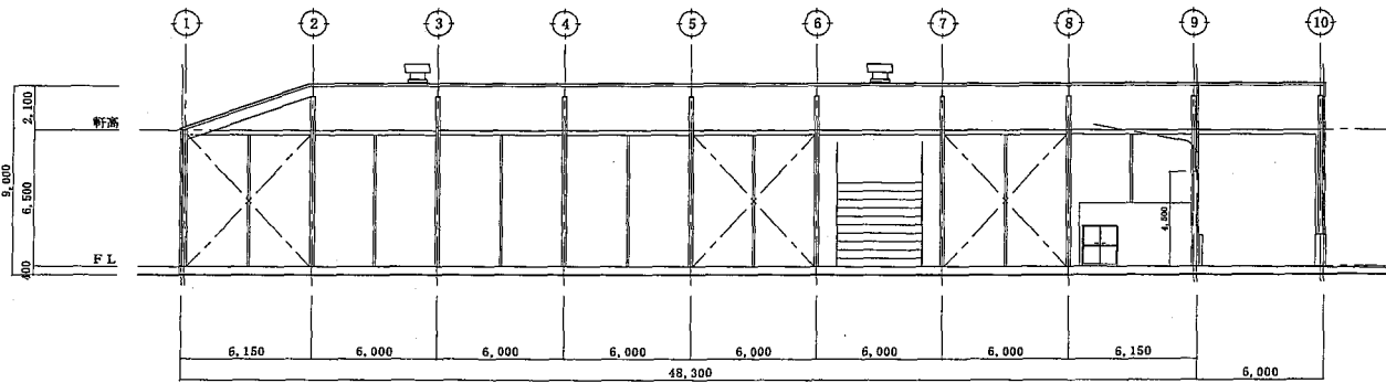
断面図 1: 200
