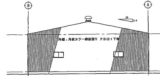
北側立面図 1: 200
