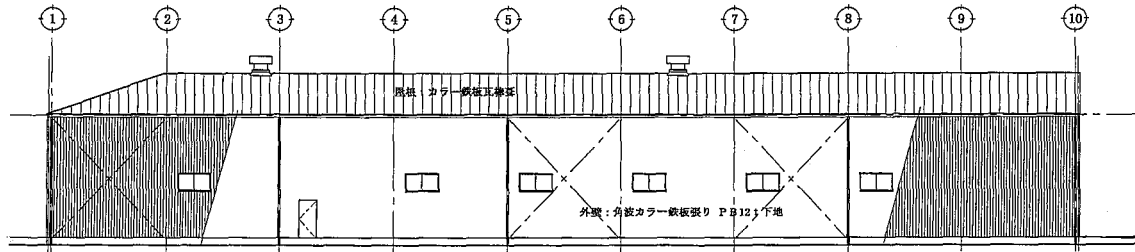
西側立面図 1: 200
