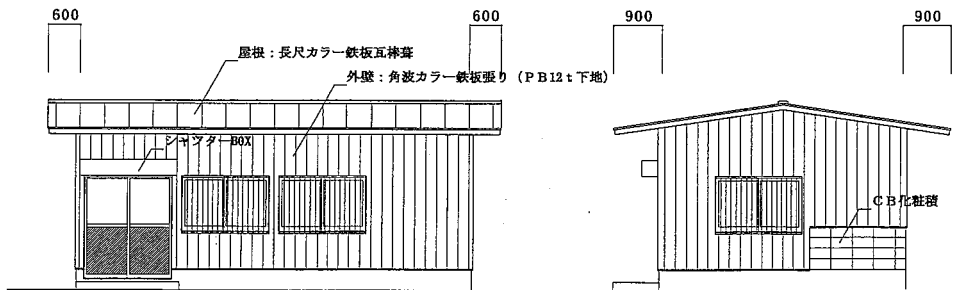
南側立平面図 S 1:100
