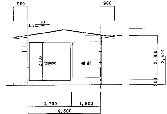
断面図 S 1:100
