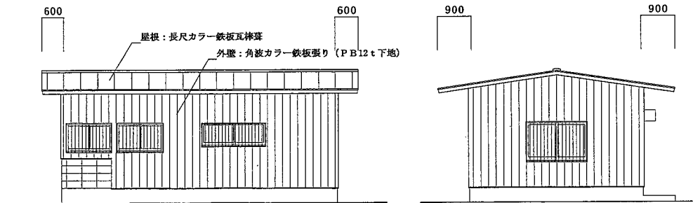
北側立平面図 S 1:100
