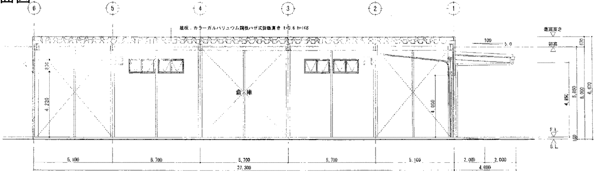
X-X 断面図 S 1:100
