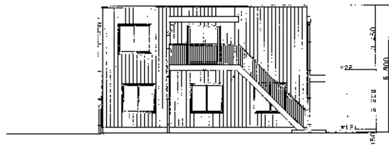
西立面図 S1:100
